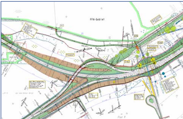
Lageplan Entwurfsplanung:
